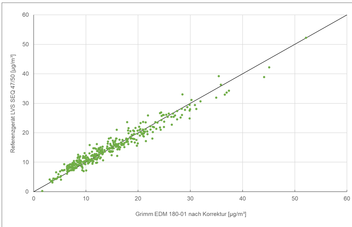
Abbildung 3: Vergleich der Wertepaare zwischen Referenzverfahren (LVS SEQ47/50) und automatischer Messung (Grimm EDM180-01) am Standort Magdeburg/Guericke-Straße.
